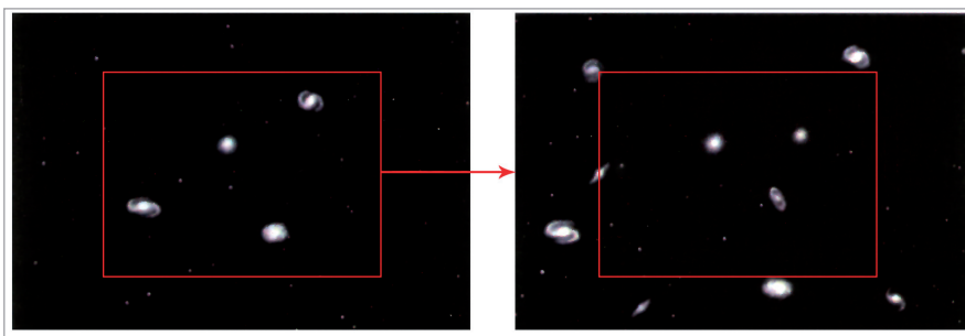
► Ez a kép azt mutatja, hogy a távolság a galaxisok vagy galaxiscsoportok között folyamatosan nő, tehát az univerzum tágul.
