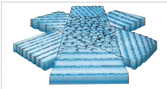
► A belső hullámok határfelületekét különböző sűrűségű vígréteg között. Az egyik sűrű (az alsó), a másik kevésbé sűrű (a felső). (Gross, Óceánográfia , 204. old.)
