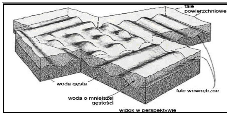
Ryc. 16: Fale wewnętrzne na styku pomiędzy dwiema warstwami wody o różnych gęstościach. Jedna jest gęsta (niższa), druga mniej gęsta (wyższa). ( Oceanography , Gross, str. 204).
