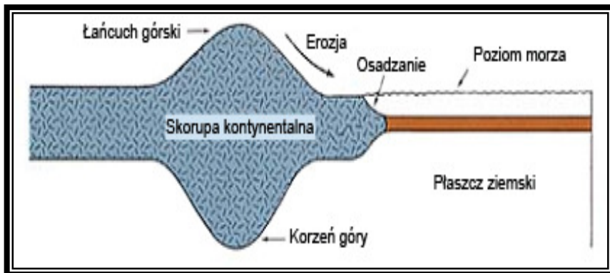
Ryc. 7: Góry mają głębokie korzenie pod powierzchnią ziemi ( Earth , Press i Siever, str. 413)
