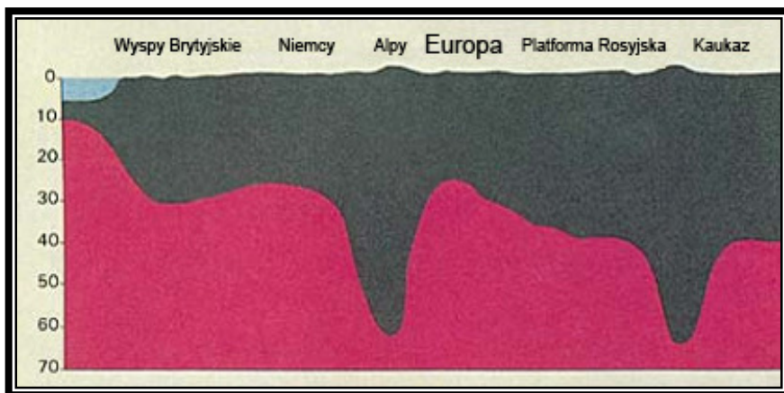
Ryc. 8: Schematyczny przekrój. Góry, jak paliki, mają głębokie korzenie pod ziemią. ( Anatomy of the Earth , Cailleux, str. 220).
