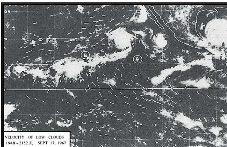
Ryc. 17: Zdjęcie satelitarne, pokazujące przesuwanie się chmur w kierunku obszarów skupiania B, C i D. Strzałki wskazują kierunek wiatru. ( The Use of Satellite Pictures in Weather Analysis and Forecasting , Anderson i inni, str. 188).
