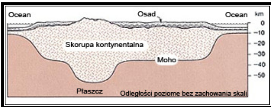
Ryc. 9: Inna ilustracja pokazująca palikowaty kształt gór, jaki nadają im głębokie korzenie. ( Earth Science , Tarbuck i Lutgens, str. 158).
