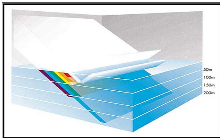
Ryc. 15: Od 3 do 30 procent promieni słonecznych odbija się od powierzchni morza. Potem prawie wszystkie z siedmiu kolorów widma światła są absorbowane, jeden po drugim, w pierwszych 200 metrach, z wyjątkiem światła niebieskiego. ( Oceans , Elder i Pernetta, str. 27).
