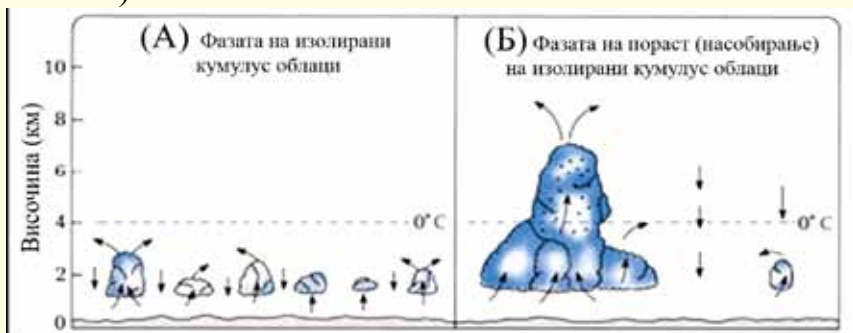
Слика 19: (А) Изолирани мали парченца облаци (кумулус облаци). (Б) Кога мали облаци се здружат заедно, движењата се зголемуваат одоздола нагоре внатре во поголемиот облак, така што облакот се насобира. Капките на водата се означени со \cdot . ( The Atmosphere, Anthes и други, стр.269 )
