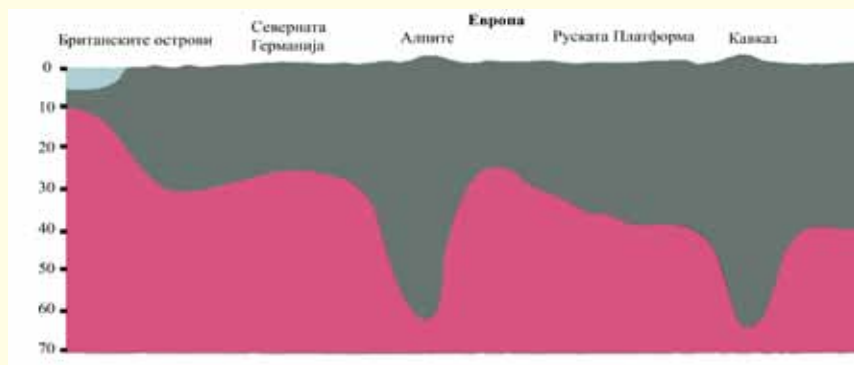
Слика 8: Шематски состав. Планините, како колчиња, имаат длабоки корени вградени во земјата. (Anatomy of the Earth, Cailleux, стр. 220.)
