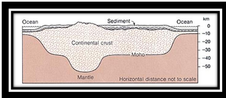
Figur 7: Fjellene har dype røtter under jordens overflate. ( Earth [Jorden], Press og Siever, s. 413).
