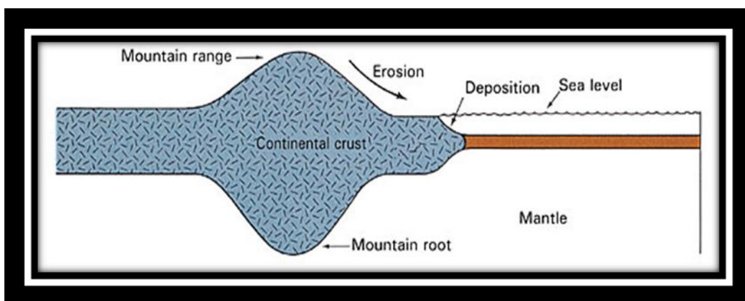
Figur 9: Denne illustrasjonen viser hvordan fjellene på grunn av de dype røttene, har plugglignende form. ( Earth Science [Vitenskapen om jorden], Tarbuck og Lutgens, s. 158).
